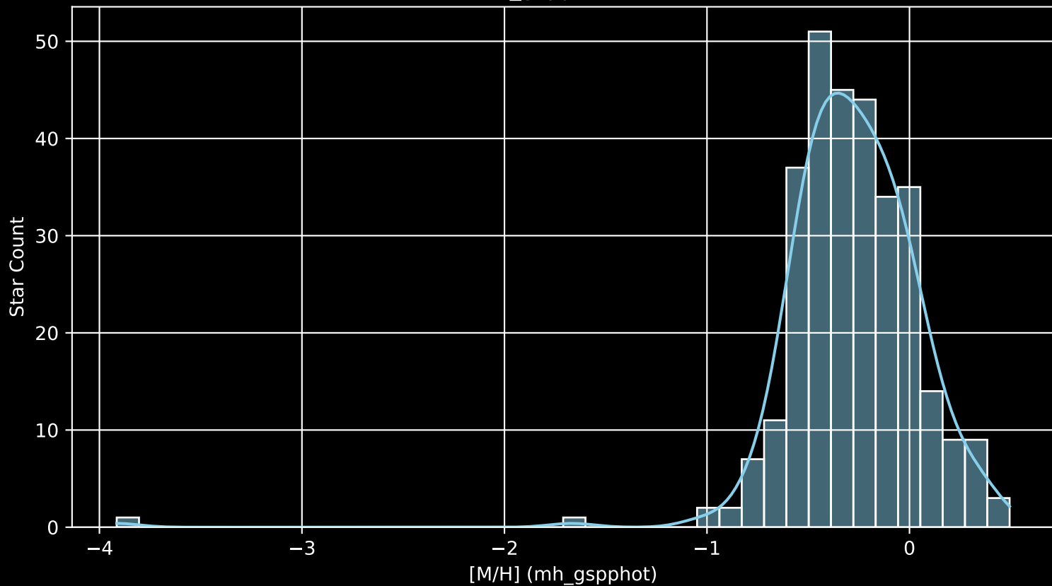
GALAH DR4 Field: [397] [M/H] (mh_gspphot) (n= 305)
