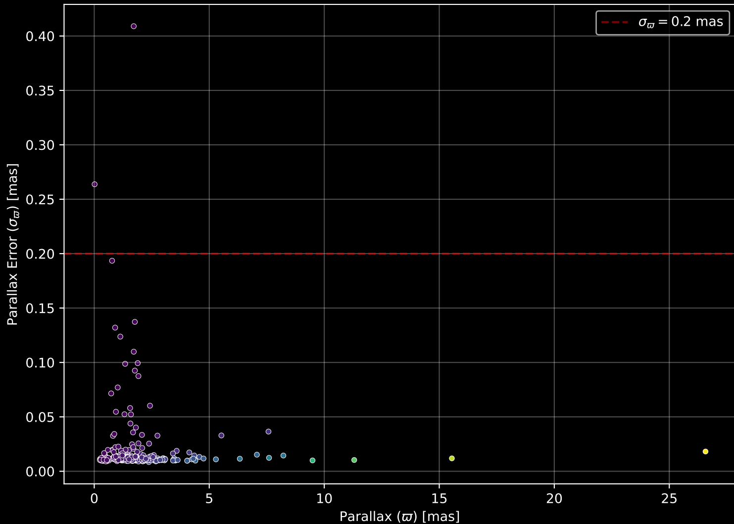
GALAH DR4 Field: [397] Parallax Quality (n= 305)
