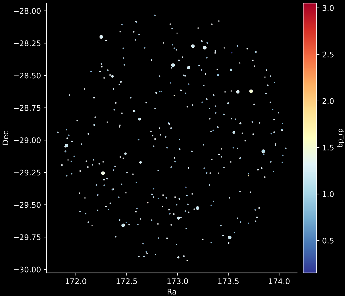
GALAH DR4 Field: [397] Stars: 305
