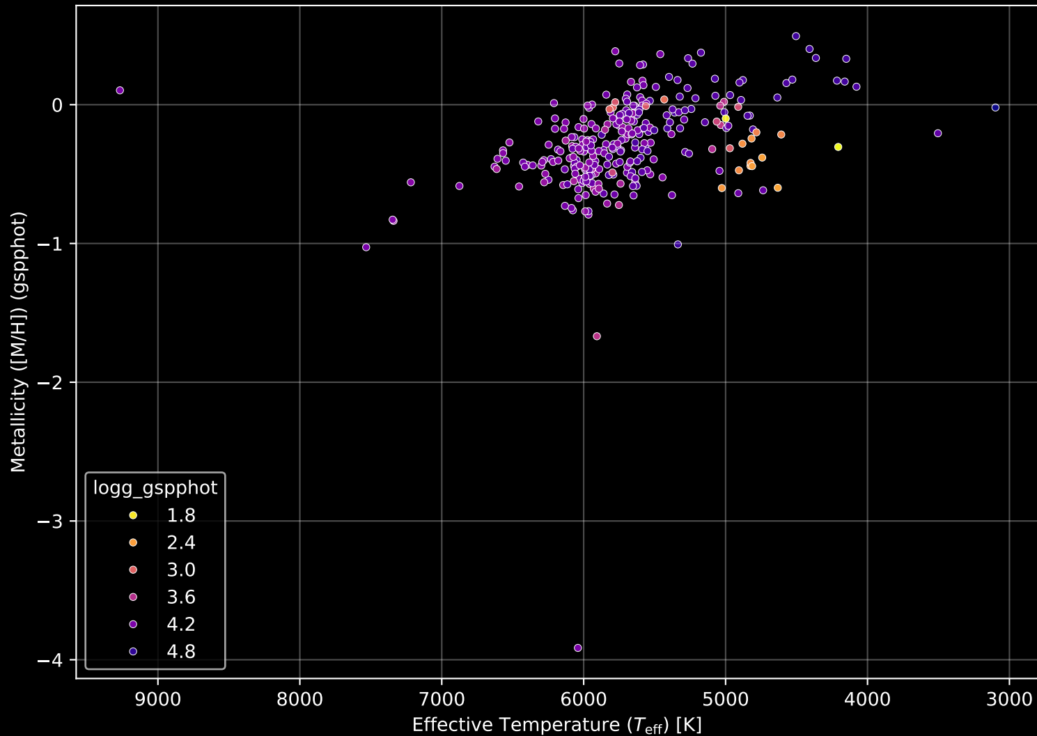
GALAH DR4 Field: [397] Stellar Population Parameters (n= 305)
